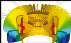
Skupiony przepływ powietrza Głośniki podczas pracy rozgrzewają się. Może powodować to drastyczne spadki mocy i jakości dźwięku podczas długiej pracy. Nasz opatentowany system Ram Air Cooling skupia przepływ powietrza na zewnątrz głośnika, zapewniając najlepsze chłodzenie i perfekcyjny dźwięk.
